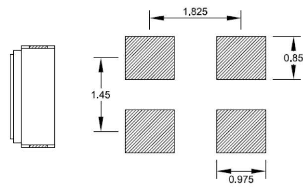
推荐焊盘图
